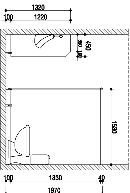
CHI TIẾT MẶT BÊN DIỆN HÌNH VÁCH NGĂN WC
